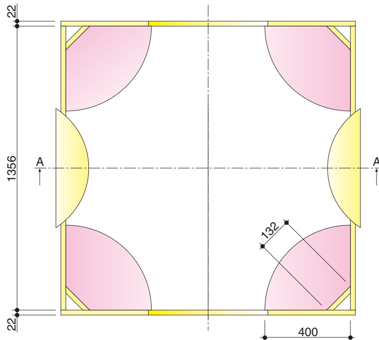
Draufsicht (ohne Dach)
