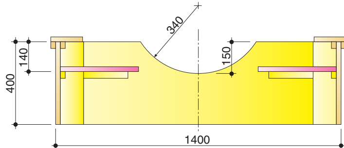
Schnitt A+A
