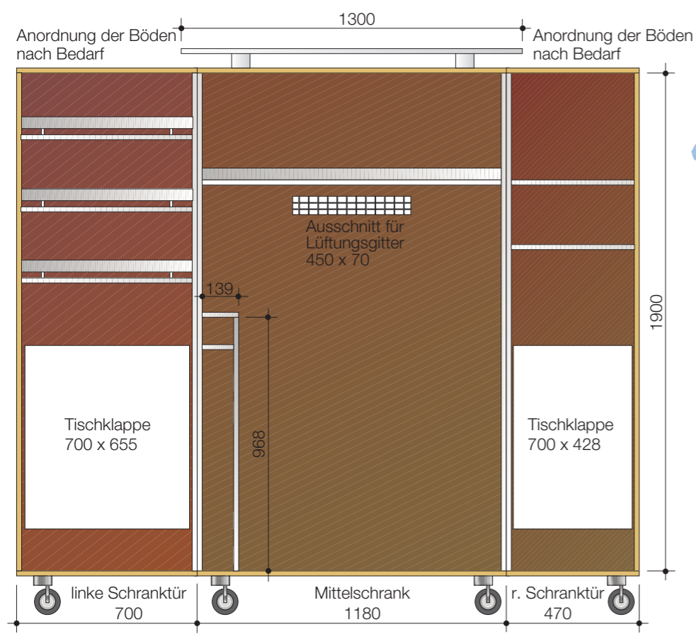
Als Wetterschutz wird ein Kunststoffdach mit Gefälle aufgesetzt. Das Dach liegt auf Distanzstücken auf und wird mit Gewindestäben, U-Scheiben und Hutmuttern von oben und unten befestigt. Ein Lüftungsgitter (siehe Zeichnung links) sorgt für Luftaustausch auch bei Nichtgebrauch. Vorderansicht des geöffneten Schanks
