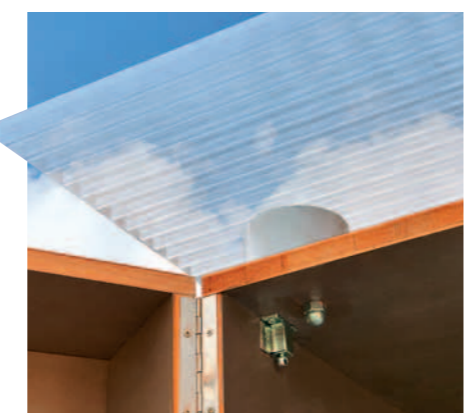
Als Wetterschutz wird ein Kunststoffdach mit Gefälle aufgesetzt. Das Dach liegt auf Distanzstücken auf und wird mit Gewindestäben, U-Scheiben und Hutmuttern von oben und unten befestigt. Ein Lüftungsgitter (siehe Zeichnung links) sorgt für Luftaustausch auch bei Nichtgebrauch. Vorderansicht des geöffneten Schanks
