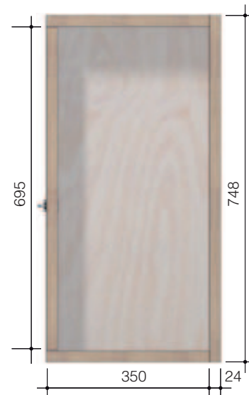
Schnitt Y - Y
