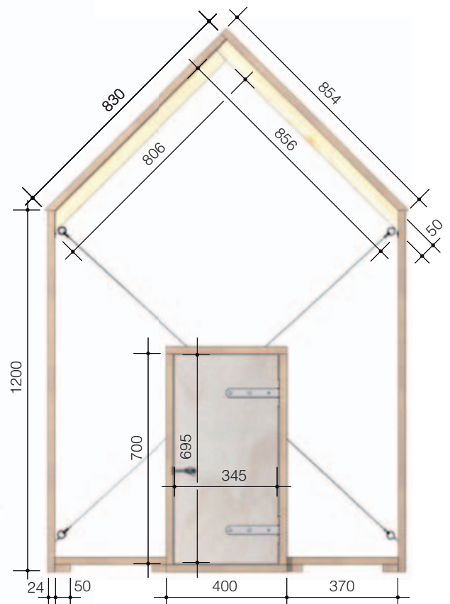
Schnitt Y - Y
