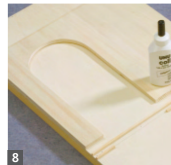
8 Für die obere Zwischenwand nur Bodenleisten, für die untere Decken- und Bodenleisten aufleimen
