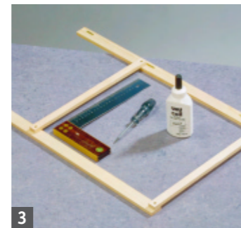
3 Nun können Sie die Rahmen mit Leim und Schrauben montieren. Achten Sie auf Rechtwinkligkeit!
